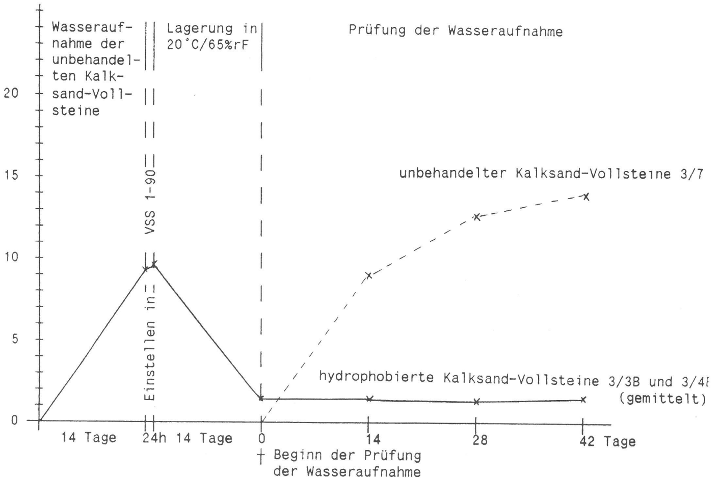
Abb. 3: Gewichtsänderungen bei der Prüfung der Wasseraufnahme von Kalksand-Vollsteinen vor und nach dem Hydrophobieren mit VSS 1-90.
