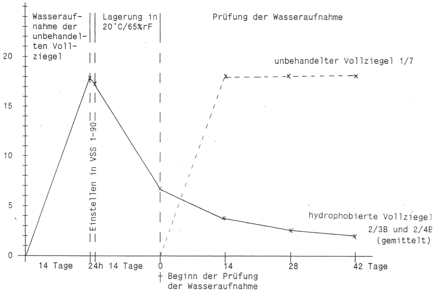
Abb. 2: Gewichtsänderungen bei der Prüfung der Wasseraufnahme von Vollziegeln vor und nach dem Hydrophobieren mit VSS 1-90.
