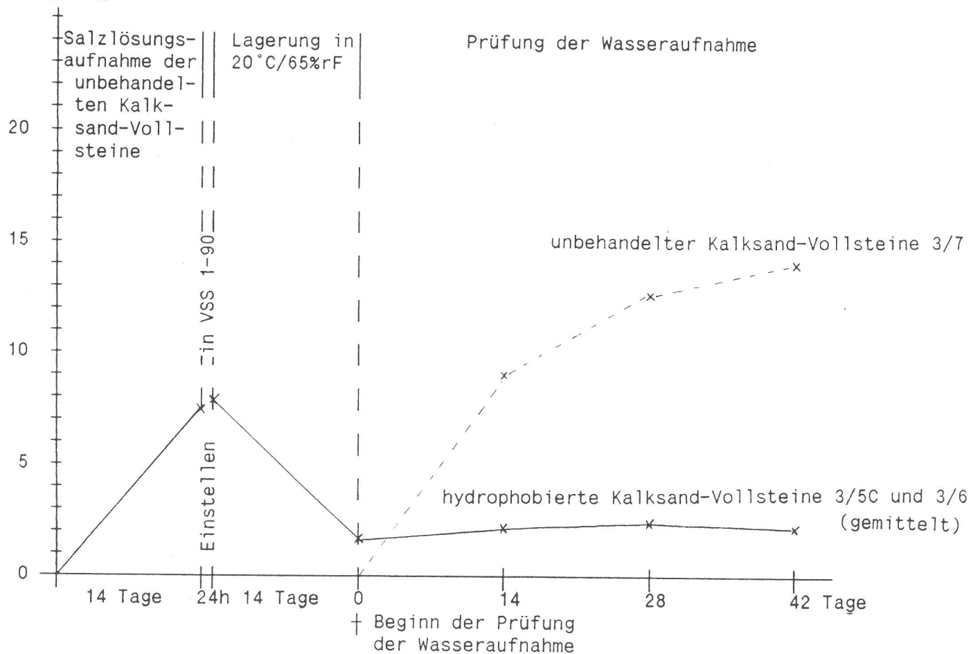
Abb. 6: Gewichtsänderungen bei der Prüfung der Salzlösungsaufnahme von Kalksand-Vollsteinen vor und nach dem Hydrophobieren mit VSS 1-90 (1%ige Salzlösung \text{NaCl} + \text{NaNO}_3 + \text{Na}_2\text{SO}_4 ).
