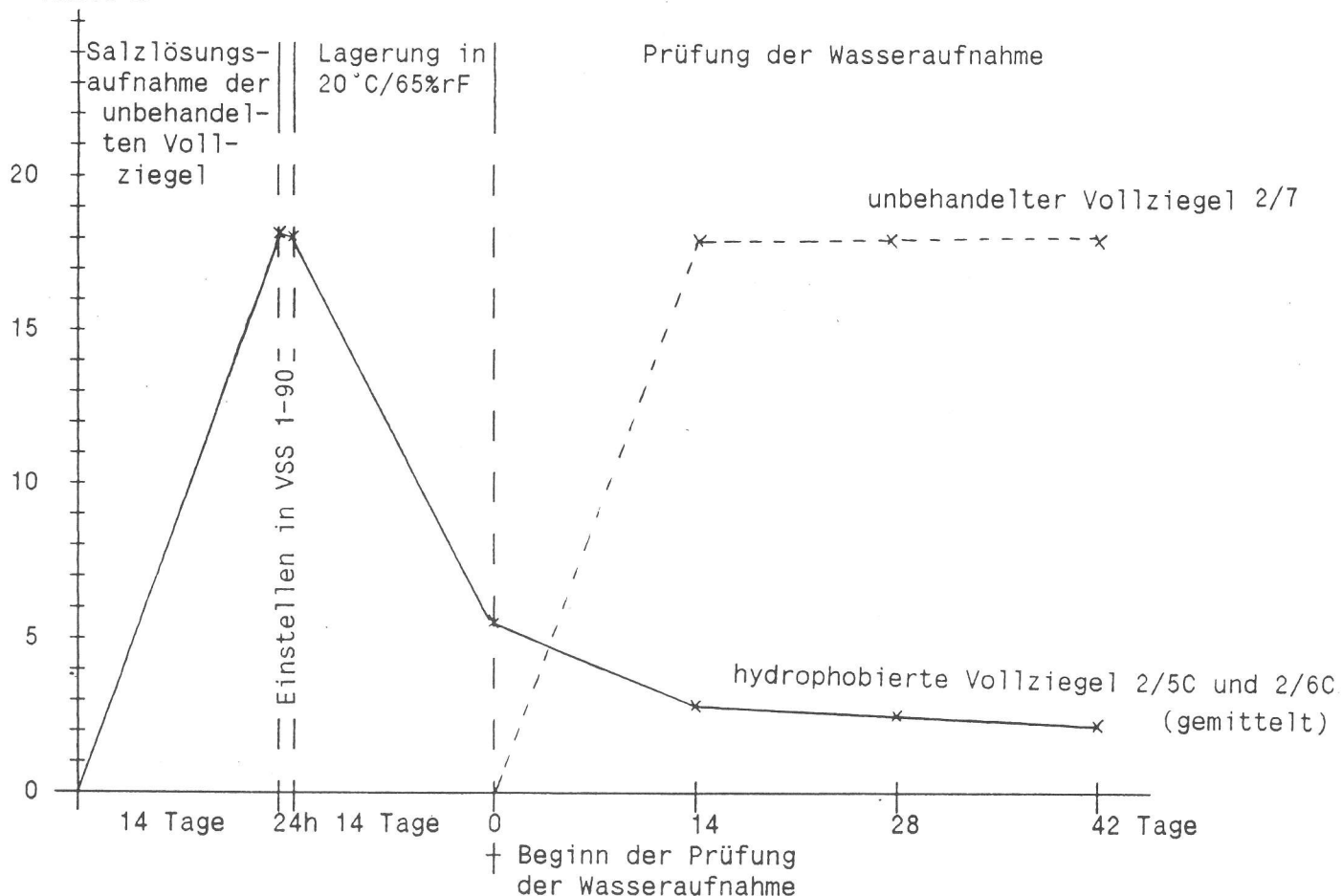
Abb. 5: Gewichtsänderungen bei der Prüfung der Salzlösungsaufnahme von Vollziegeln vor und nach dem Hydrophobieren mit VSS 1-90 (1%ige Salzlösung \text{NaCl} + \text{NaNO}_3 + \text{Na}_2\text{SO}_4 ).
