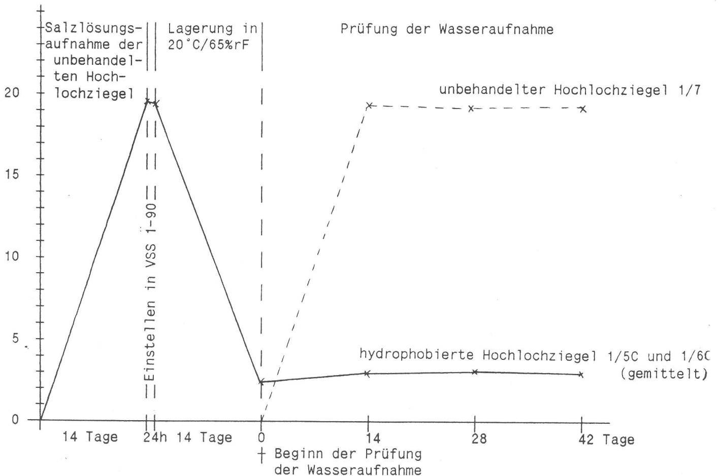
Abb. 4: Gewichtsänderungen bei der Prüfung der Salzlösungsaufnahme von Hochlochziegeln vor und nach dem Hydrophobieren mit VSS 1-90 (1%ige Salzlösung \text{NaCl} + \text{NaNO}_3 + \text{Na}_2\text{SO}_4 ).
