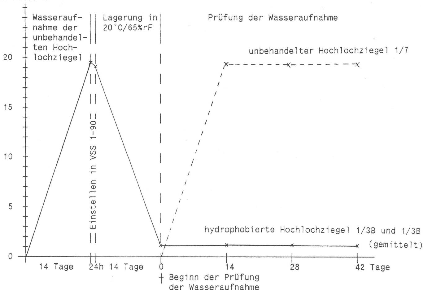
Abb. 1: Gewichtsänderungen bei der Prüfung der Wasseraufnahme von Hochlochziegeln vor und nach dem Hydrophobieren mit VSS 1-90.
