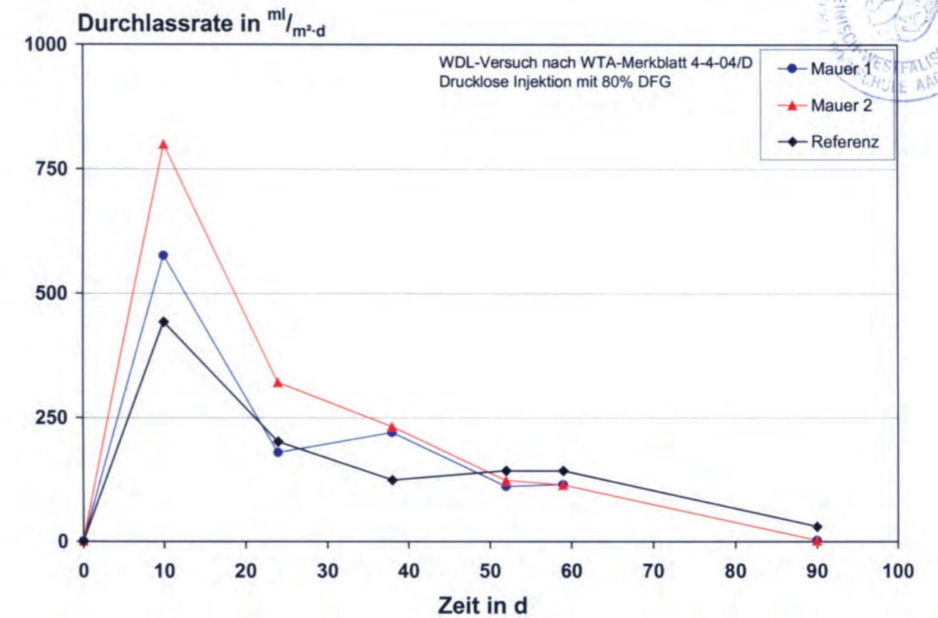
Bild B2: Wirksamkeitsprüfung an den Mauerwerken 1 und 2
